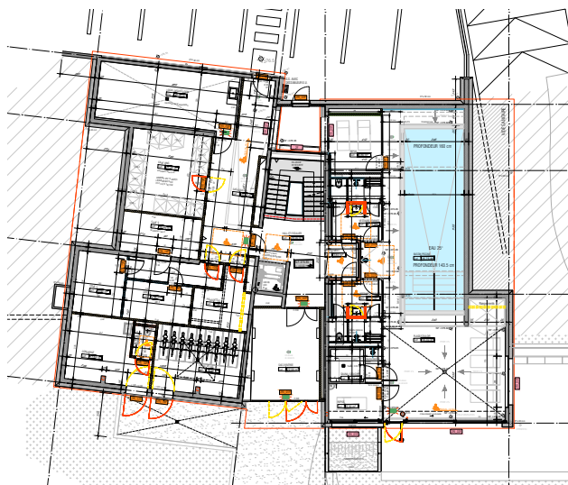
Rez inférieur
