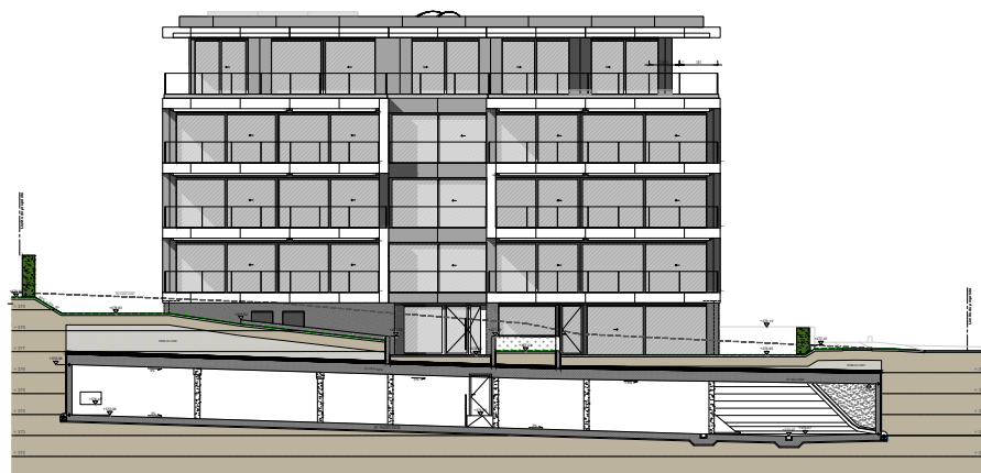
Façade sud
