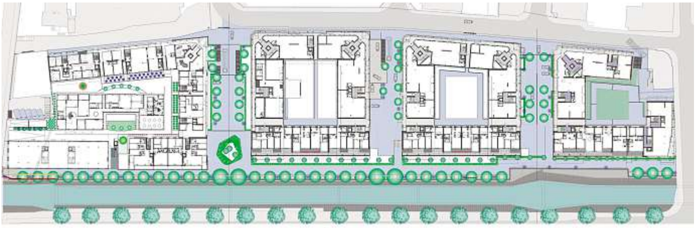
Plan ilots A+B+C+D niveau 0
